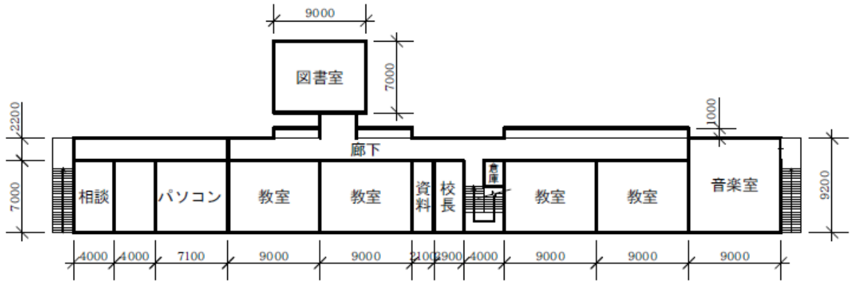
【2階平面図】
