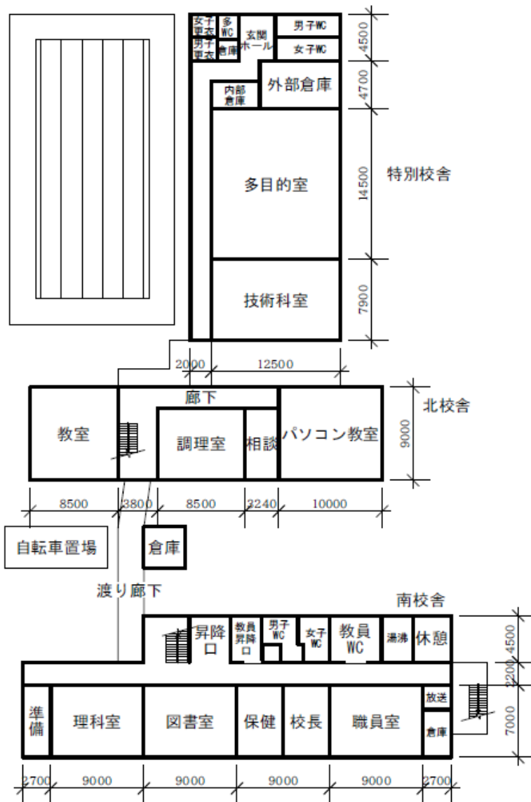
【1階平面図】
