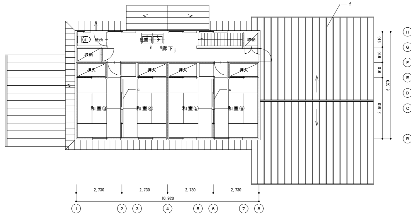
2階平面図(改修) S=1/100
