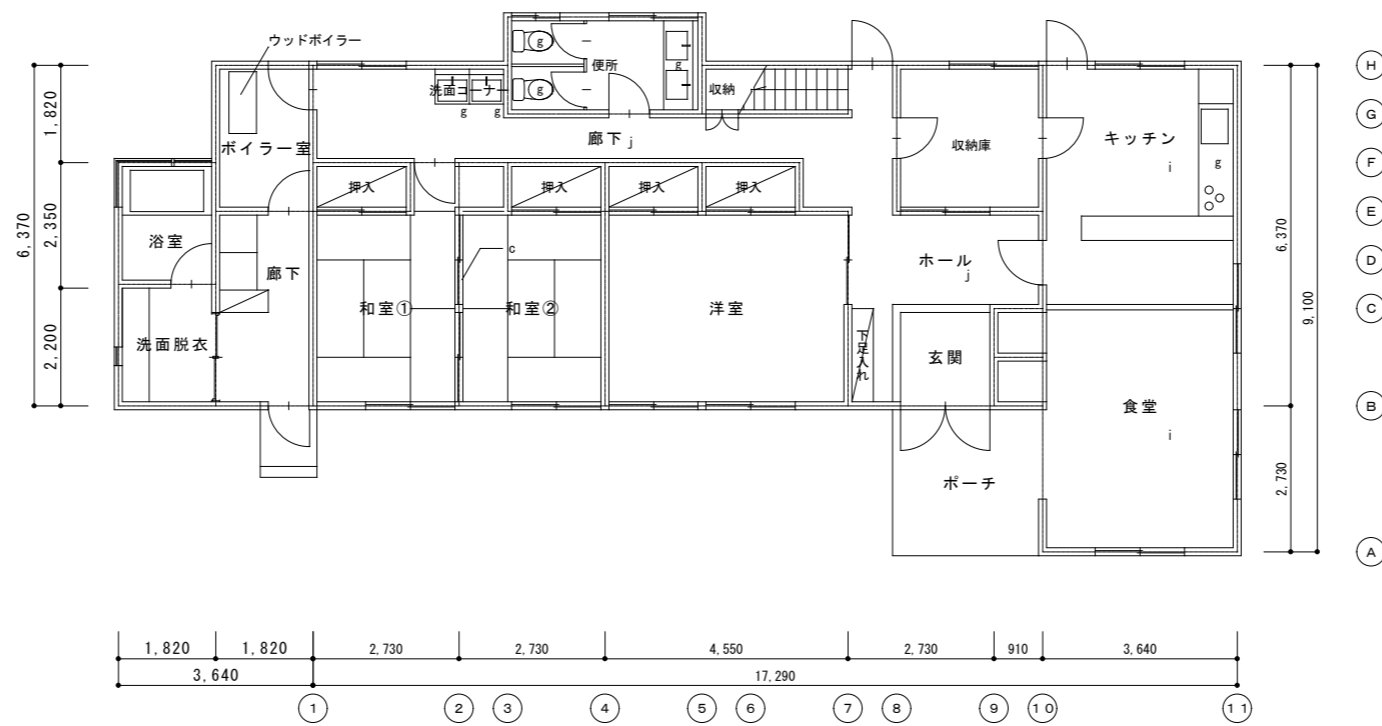
1階平面図(改修) S=1/100
